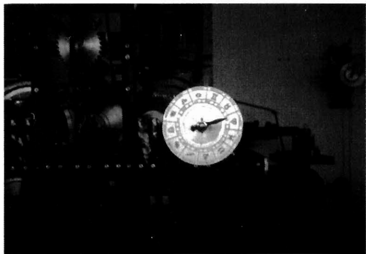
Il particolare del quadrante zodiacale
