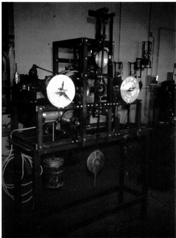
L'insieme della "macchina del tempo" di Grazie
